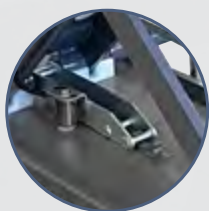
Verrouillage de la crémaillère électrique, pas besoin d'alimentation pneumatique
